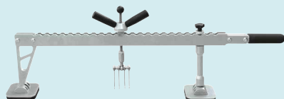
Barra per riparazione ammaccature doppia azione ref. 053564
